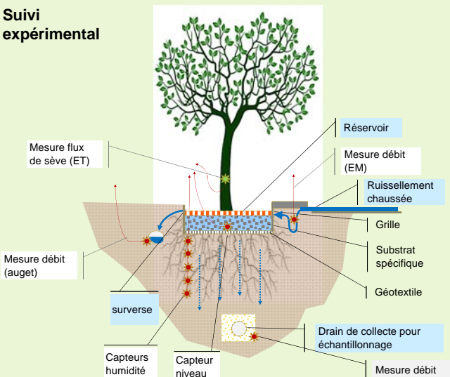
Figure 1: Mise en place expérimental des arbres de pluie.
