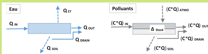
Figure 2: Les bilans à étudier. Q: débit, C: concentration
